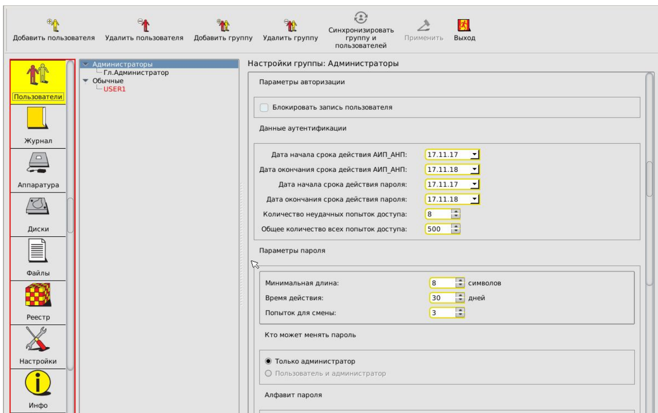
Рисунок 15 - Общие параметры группы «Администраторы» (для моделей Аккорд-АМДЗ» ТУ 4012-054-11443195-2013)
