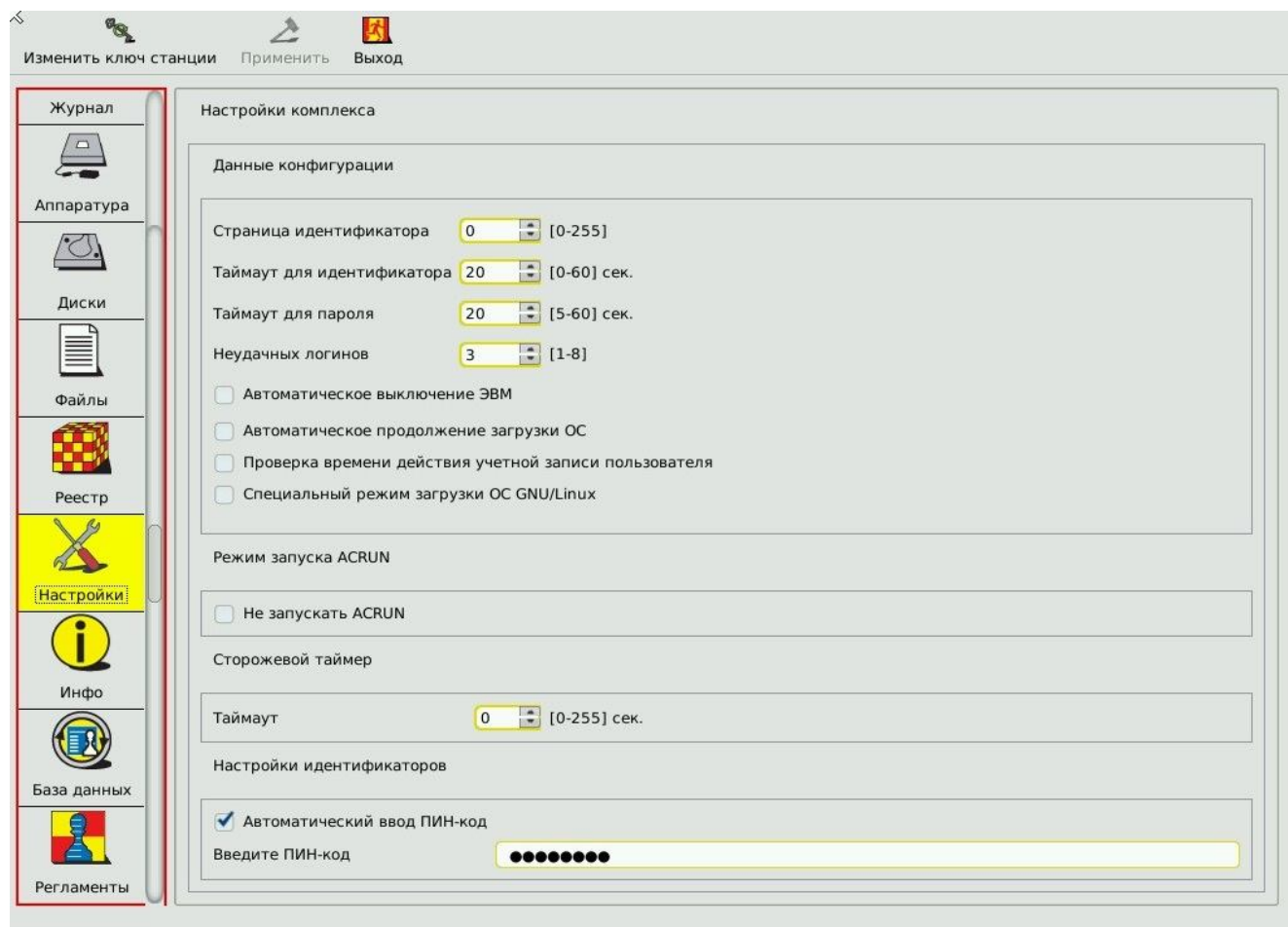
Рисунок 36 - Общие настройки комплекса (для моделей «Аккорд-АМД3 ТУ 4012-054-11443195-2013»)
