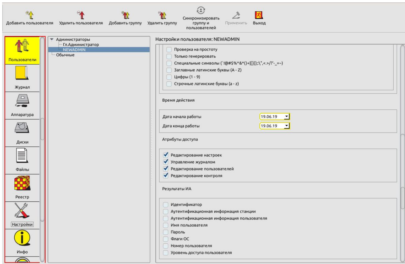
Рисунок 20 – Атрибуты доступа для пользователей из группы «Администраторы»
