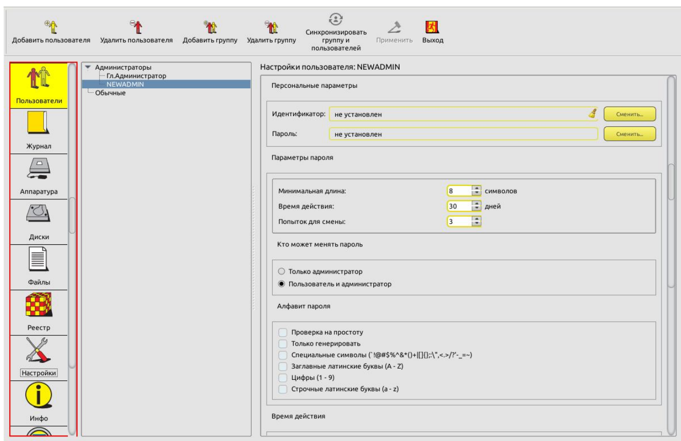
Рисунок 18 – Параметры пользователей в группе «Администраторы» (для моделей Аккорд-АМДЗ» ТУ 4012-038-11443195-2011 и ТУ 26.20.40.140-079-37222406-2019)
