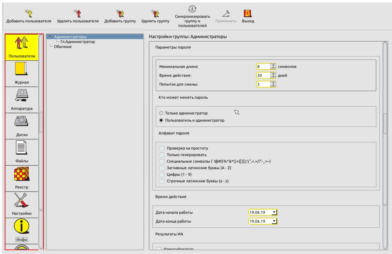
Рисунок 14 - Общие параметры группы «Администраторы» (для моделей Аккорд-АМДЗ» ТУ 4012-038-11443195-2011 и ТУ 26.20.40.140-079-37222406-2019)
