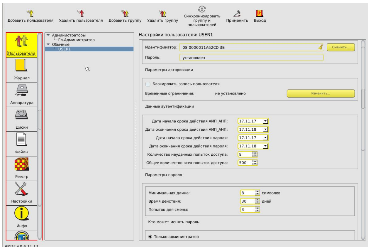
Рисунок 22 - Параметры пользователей в группе «Обычные» (для моделей Аккорд-АМДЗ» ТУ 4012-054-11443195-2013)
