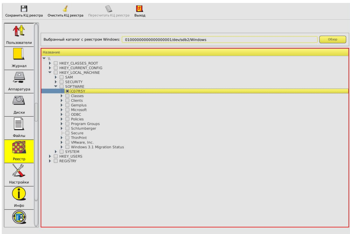
Рисунок 33 - Постановка ветви реестра на контроль целостности
