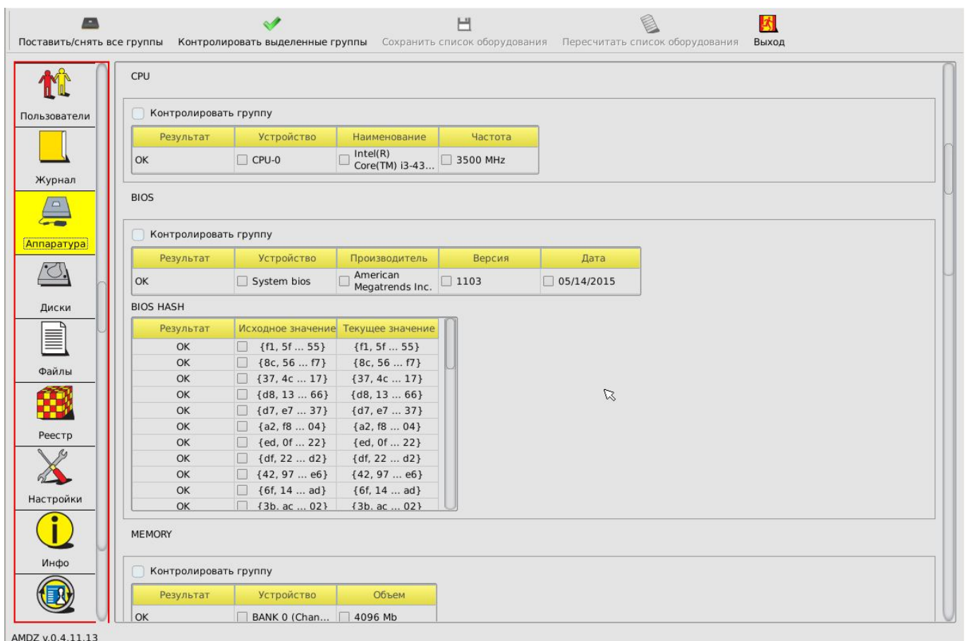
Рисунок 24 - Окно контроля аппаратной части компьютера
