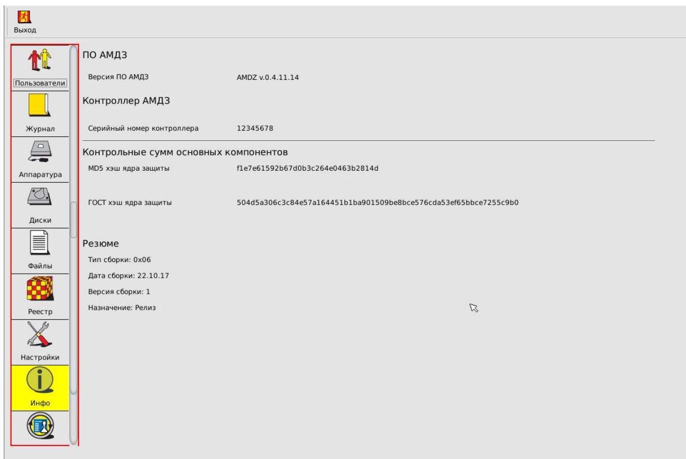
Рисунок 37 - Вкладка «Инфо» главного окна среды администрирования
