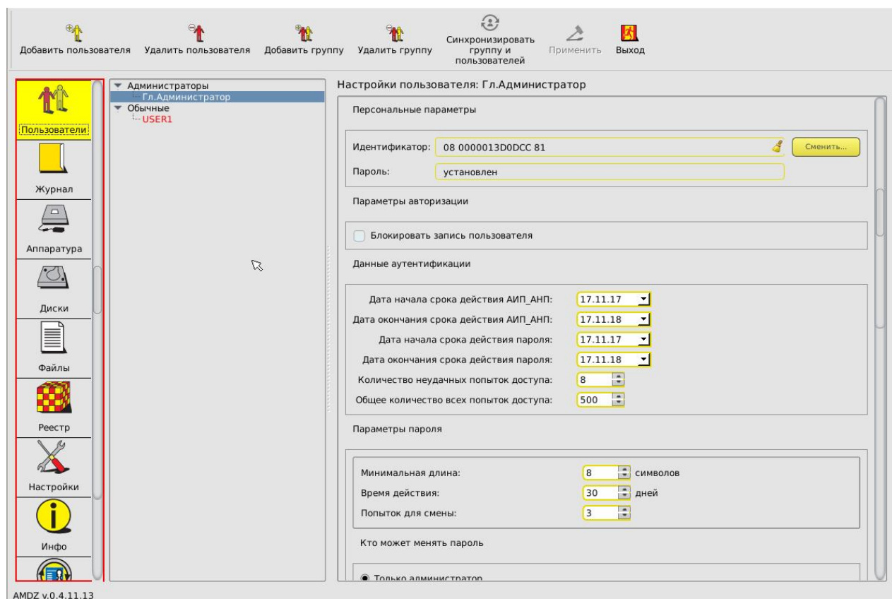
Рисунок 19 - Параметры пользователей в группе «Администраторы» (для моделей Аккорд-АМДЗ» ТУ 4012-054-11443195-2013)
