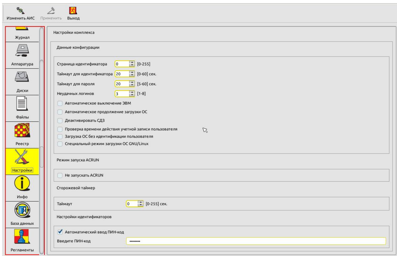
Рисунок 10 – Установка автоматического ввода ПИН-кода
