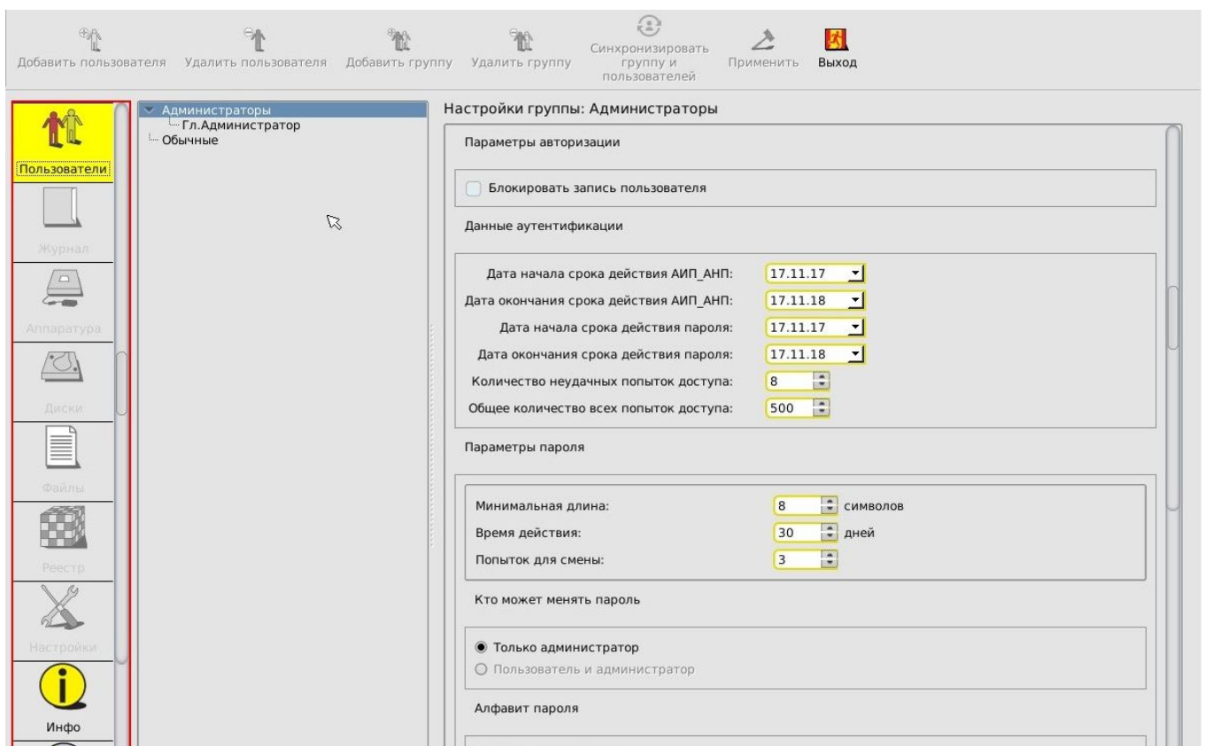
Рисунок 2 - Главное окно среды администрирования (для моделей Аккорд-АМДЗ» ТУ 4012-054-11443195-2013)
