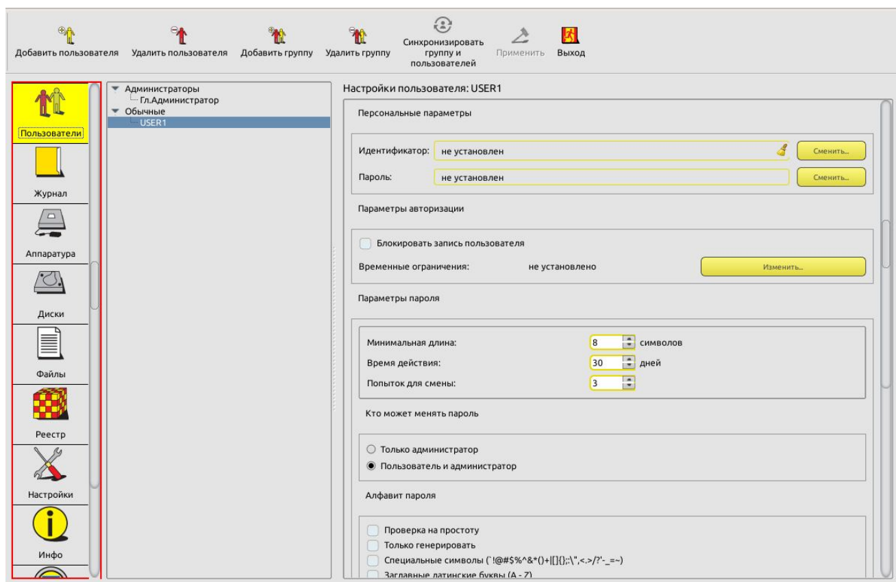
Рисунок 21 – Параметры пользователей в группе «Обычные» (для моделей Аккорд-АМДЗ» ТУ 4012-038-11443195-2011 и ТУ 26.20.40.140-079-37222406-2019)
