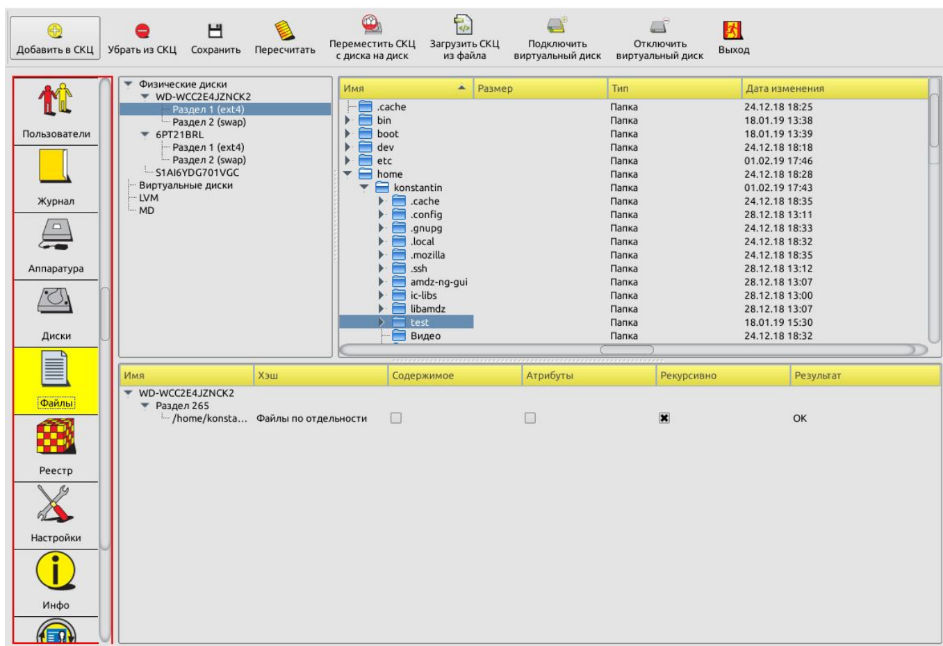
Рисунок 28 – Список контроля целостности с добавленным в него каталогом
