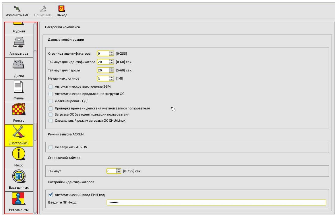
Рисунок 35 - Общие настройки комплекса (для моделей «Аккорд-АМДЗ ТУ 4012-038-11443195-2011 и ТУ 26.20.40.140-079-37222406-2019)
